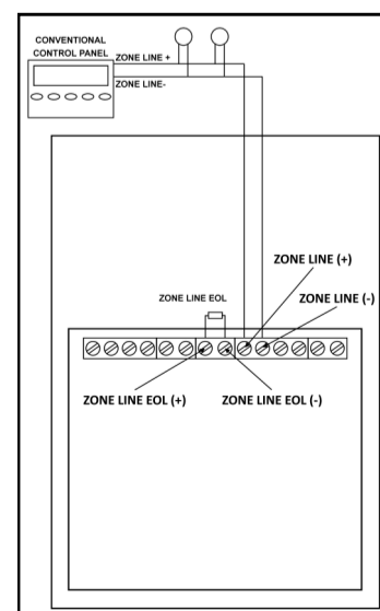
Figura 11 - Cablaggio della linea convenzionale (la resistenza EOL della linea di zona è nel dispositivo)
