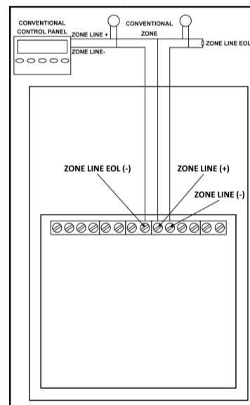
Figura 10 - Cablaggio della linea convenzionale (la resistenza EOL della linea di zona è esterna al dispositivo)
