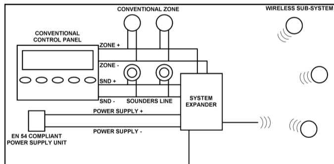
Figura 4 - Esempio di sistema radio convenzionale
