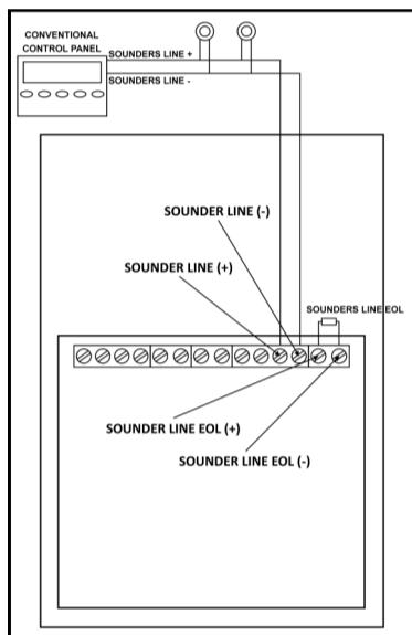
Figura 13 - Cablaggio della linea delle sirene (resistenza EOL della linea delle sirene interna al dispositivo)
