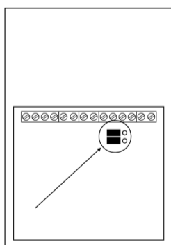
Figura 15 - Posizionamento corretto dei ponti elettrici
