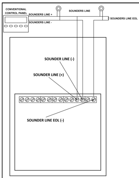
Figura 12 - Cablaggio della linea delle sirene (resistenza di fine linea EOL esterna al dispositivo)
