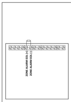
Figura 14 - Morsetti per l'installazione dell'EOL della zona di allarme
