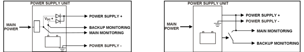
Figure 6 & 7 - Esempio di schemi di alimentazione
